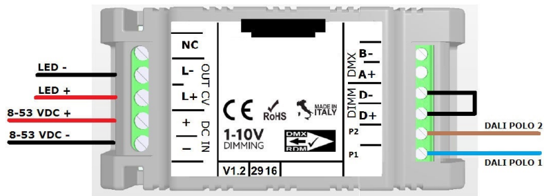
COLLEGAMENTO DALI L412MA04T1A01 - FIGURA N. 8
