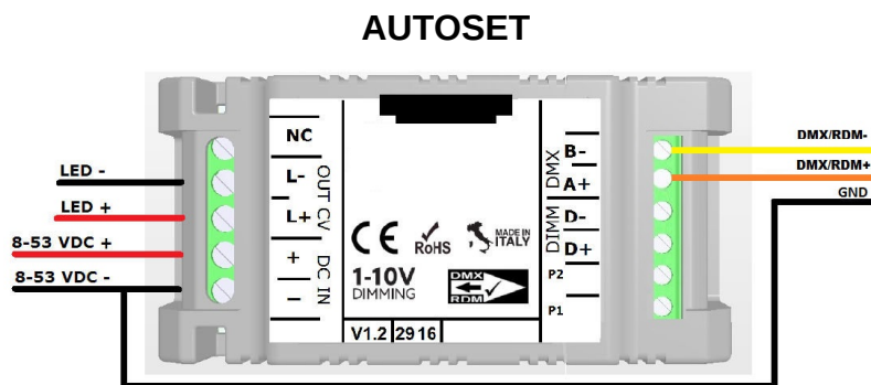
COLLEGAMENTO L412MA04T1A01 A BUS DMX512/RDM - FIGURA N. 4
