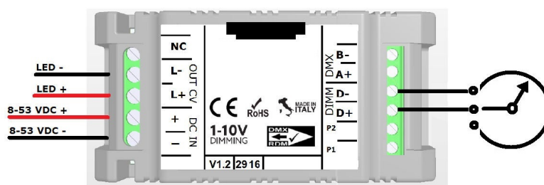
COLLEGAMENTO POTENZIOMETRO L412MA04T1A01 - FIGURA N. 6
