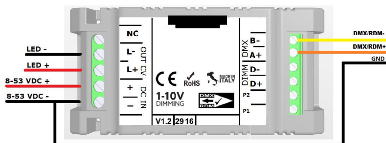
COLLEGAMENTO L412MA04T1A01 A BUS DMX512/RDM - FIGURA N. 2
