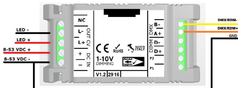
COLLEGAMENTO L412MA04T1A01 A BUS DMX512/RDM - FIGURA N. 3
