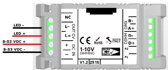
SCHEMA COLLEGAMENTO ALIMENTAZIONE E LED L412MA04T1A01 - FIGURA N. 1
