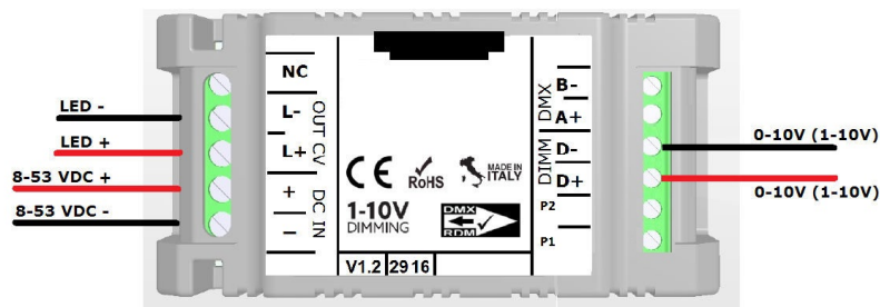
COLLEGAMENTO 0-10V L412MA04T1A01 - FIGURA N. 7
