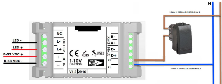
COLLEGAMENTO PULSANTE L412MA04T1A01 - FIGURA N. 5
