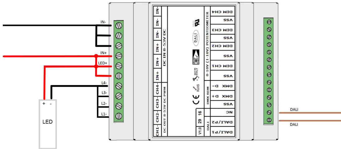
DALI WIRING DIAGRAM L406MA02T4A01 - FIGURE N. 7
