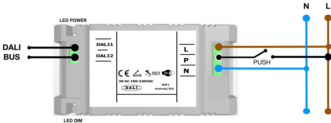
SCHEMA DI COLLEGAMENTO L607MA04D1A02 - FIGURA N. 1
